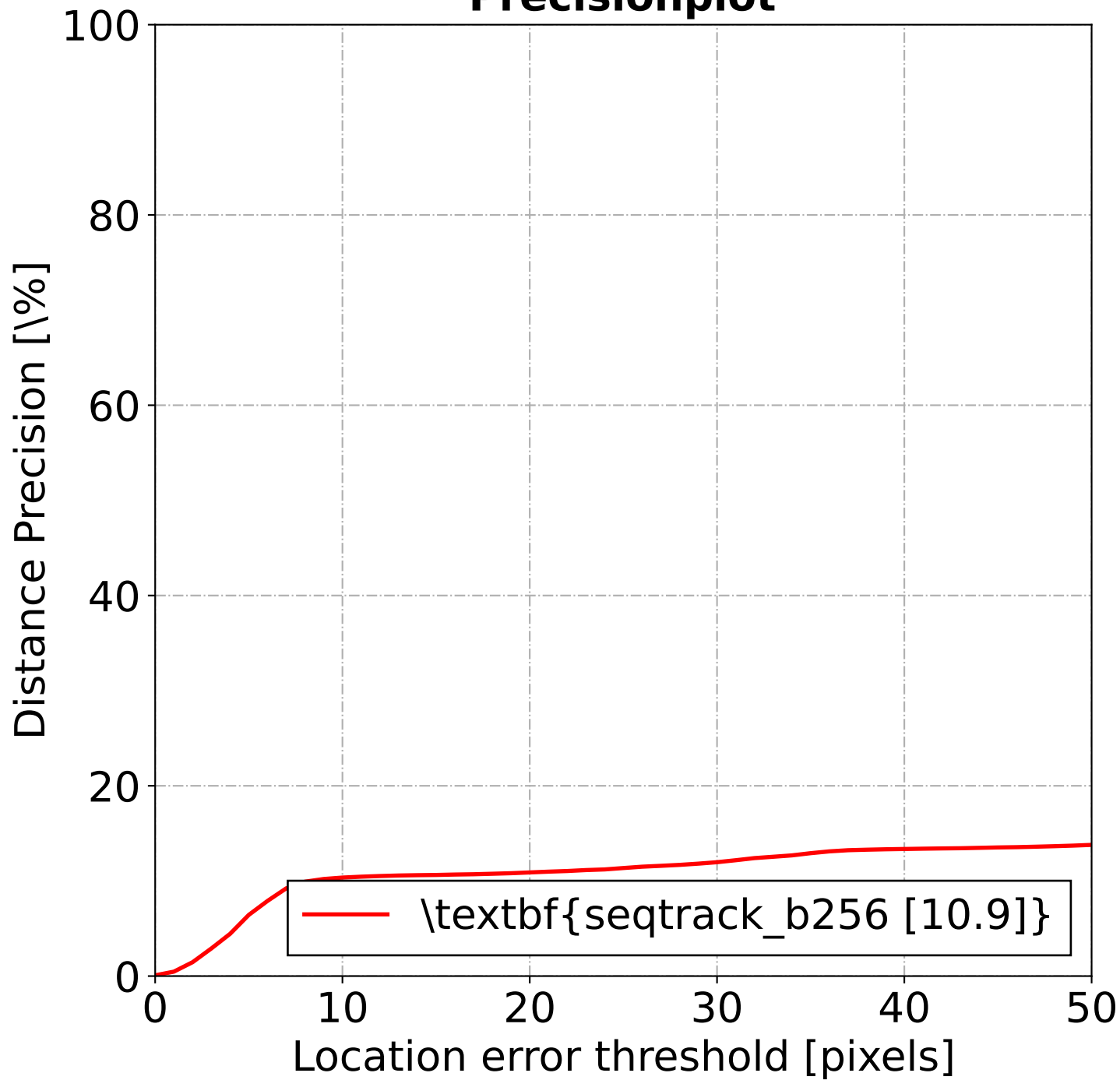
Precisionplot
